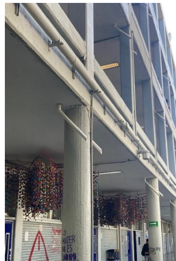
Figuras 44 y 45. Mantenimiento de bajadas de agua pluvial en edificios A y B
