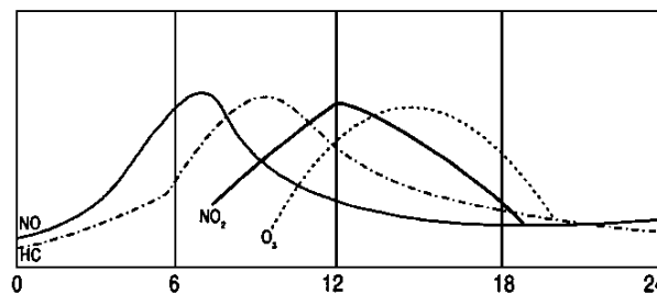
Figura 1. Evolución de la concentración de contaminantes (ppm) durante el día en el Valle de México.
